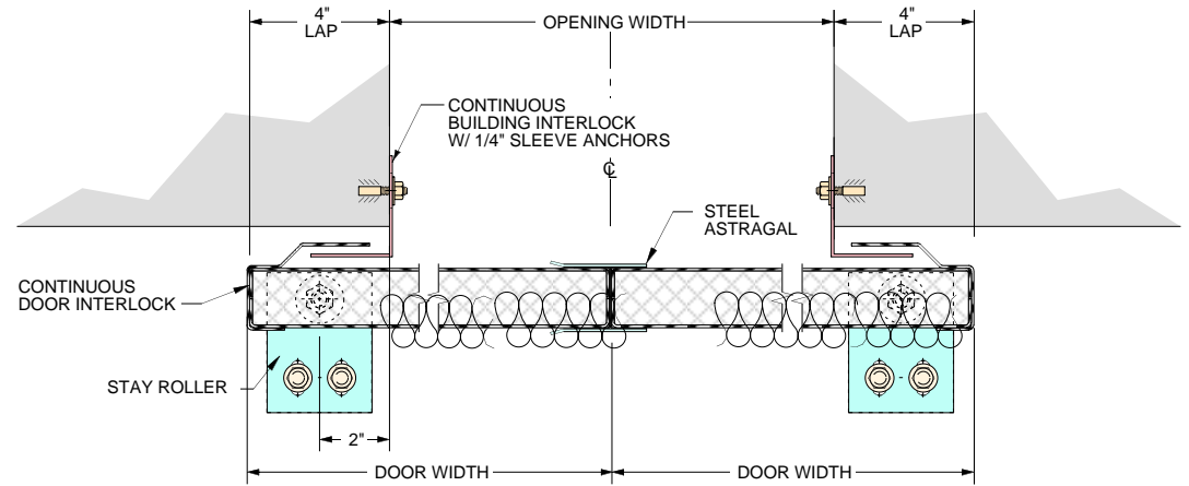
JAMB DETAIL
