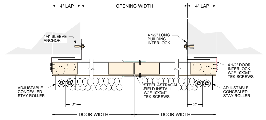
JAMB DETAIL
